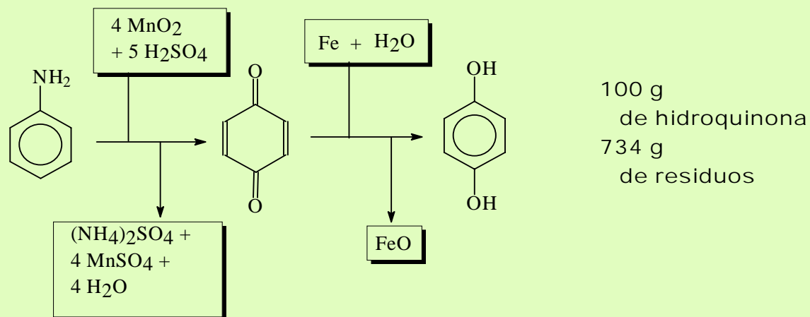
NUEVO PROCESO DE SÍNTESIS DE LA HIDROQUINONA
