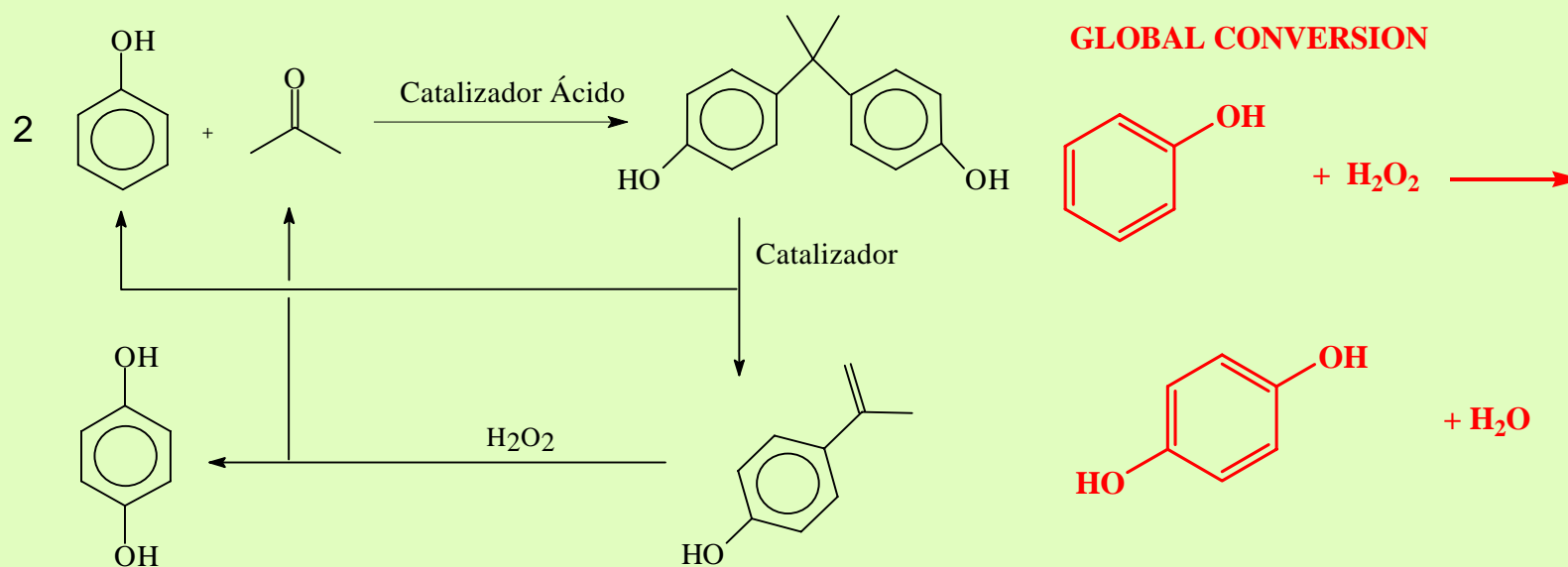
NUEVO PROCESO DE SÍNTESIS DE LA HIDROQUINONA
