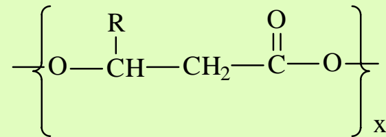
R = Me; Poli-3-hidroxitirato R = Et; Poli-3-hidroxi valerato
